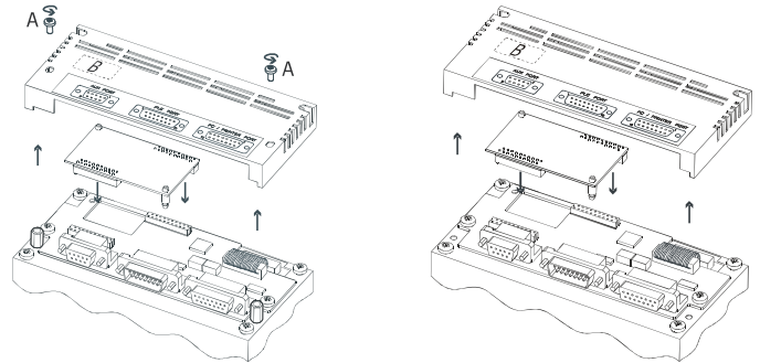
Figure 2 – Montaggio modulo porta AUX.
