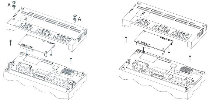
Figure 2 – Montaggio modulo porta AUX.
