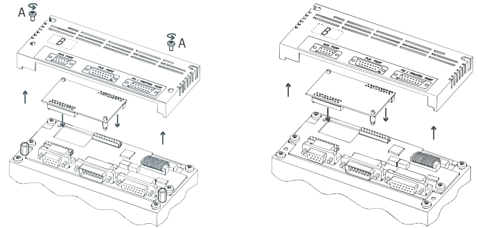
Figura 2 – Montaggio modulo SCM05.
